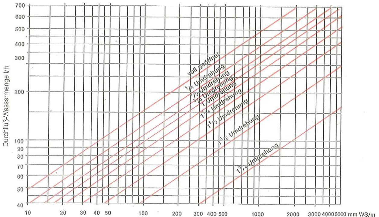
Druckverlustdiagramm für Heizkreisverteiler
