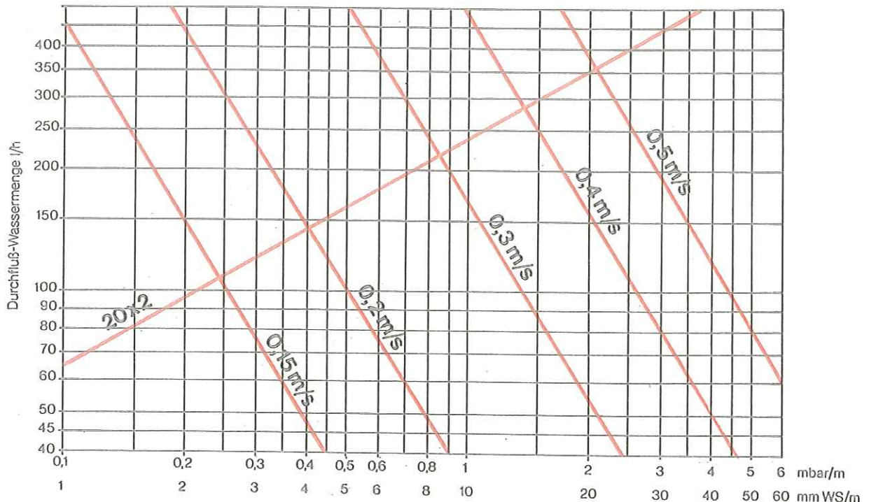
Druckverlustdiagramm für NTS-PP-C-Heizrohr 20 x 2 mm
